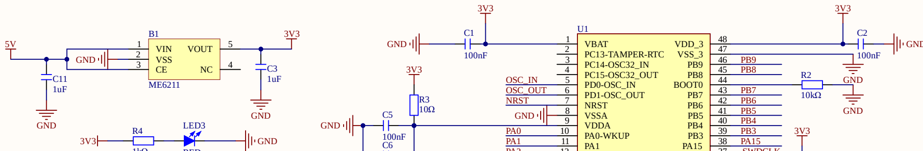
3V3稳压电路
