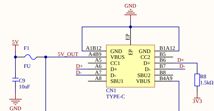
TYPEC接口电路
